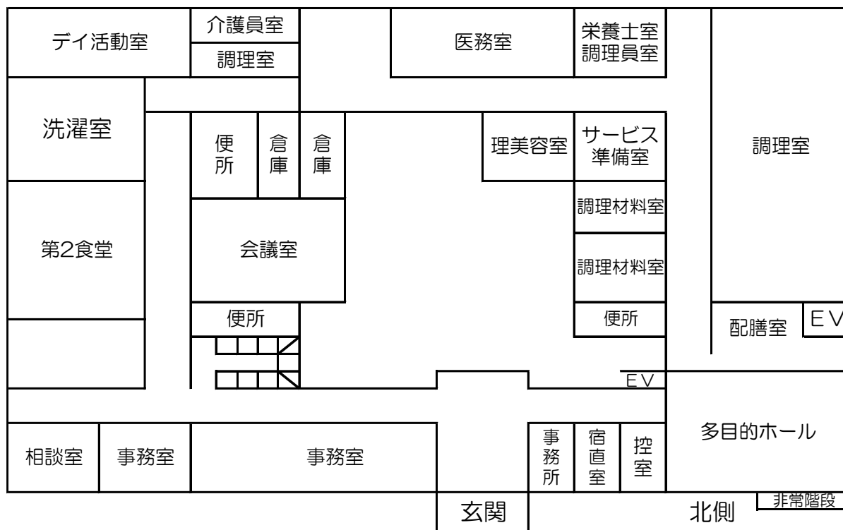
《1階 平面図》
